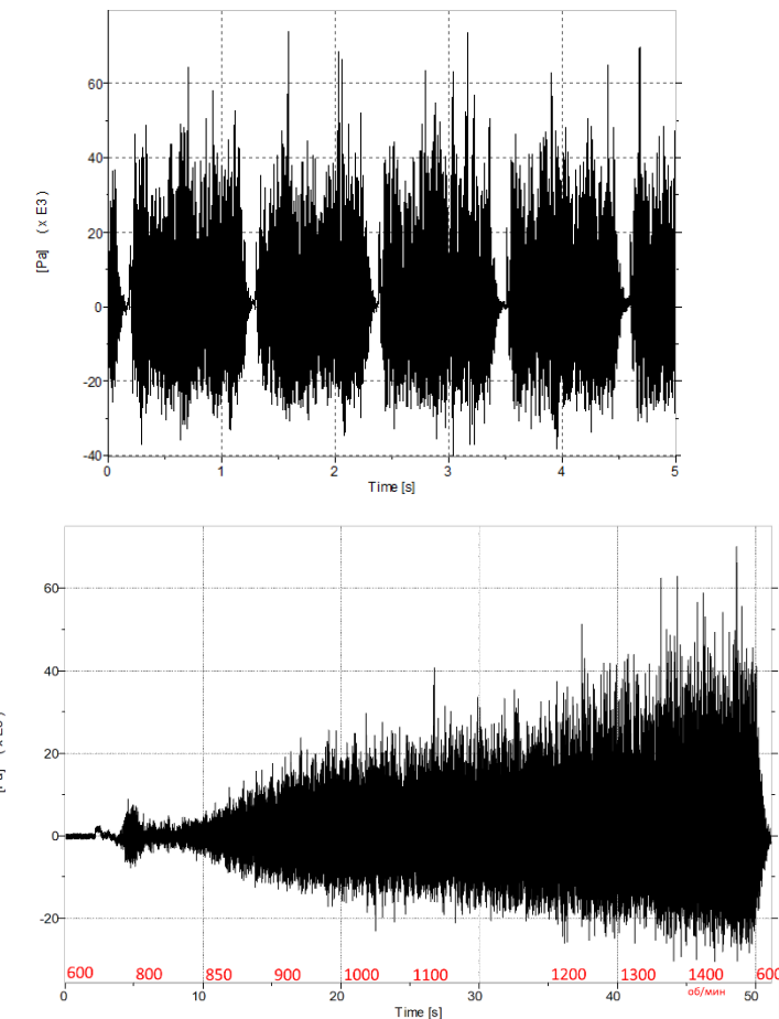
Амплитудная характеристика ГМ-88 во времени в зависимости от оборотов двигателя насосного агрегата
