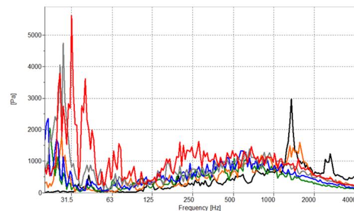
Частотно-амплитудная характеристика оборудования при расходах от 2,5 до 10 л/с
