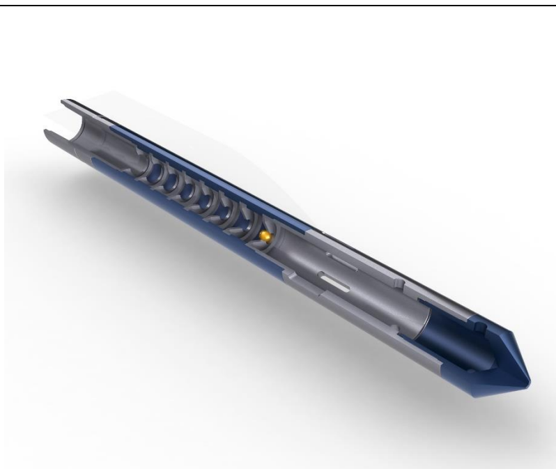
Сбрасываемый металлический шар перекрывает проходное сечение диафрагм П-94 «Геркулес»
